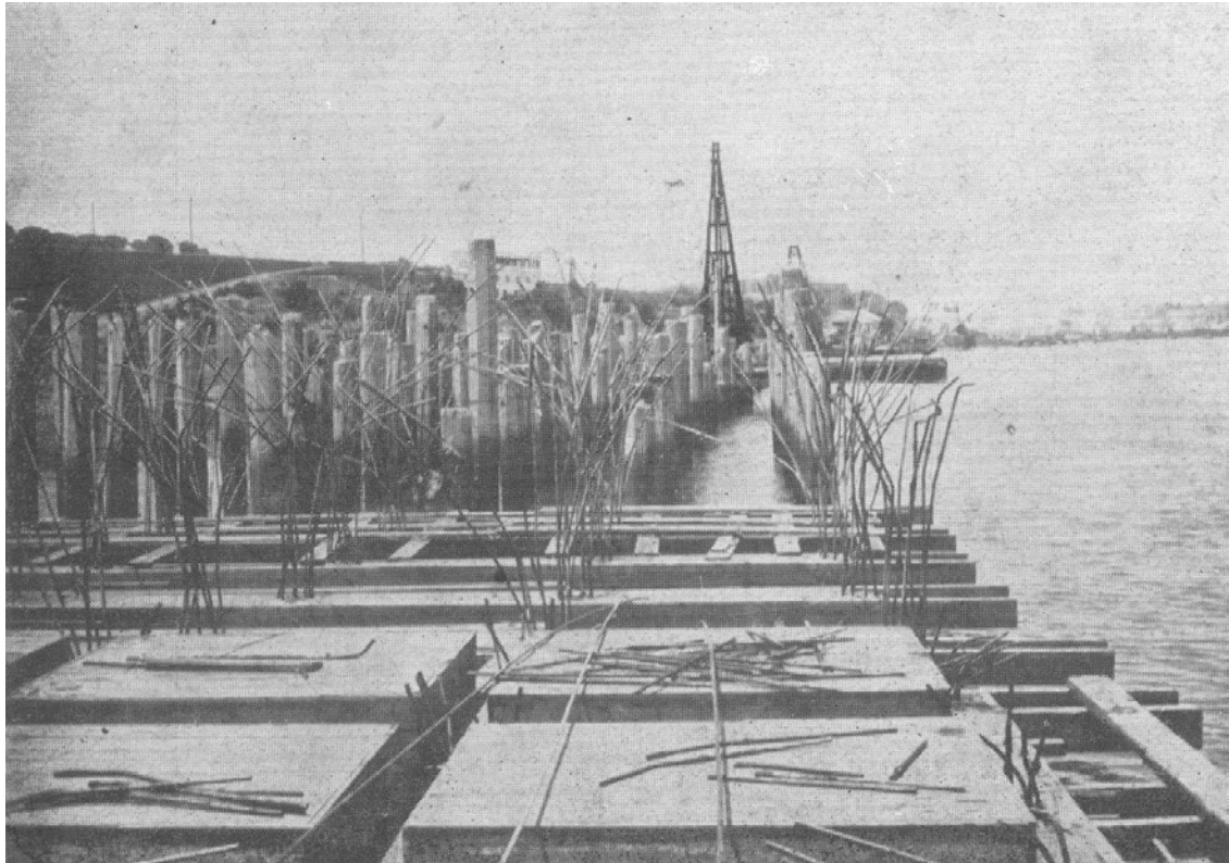
Coffrages au quai de Rabat
