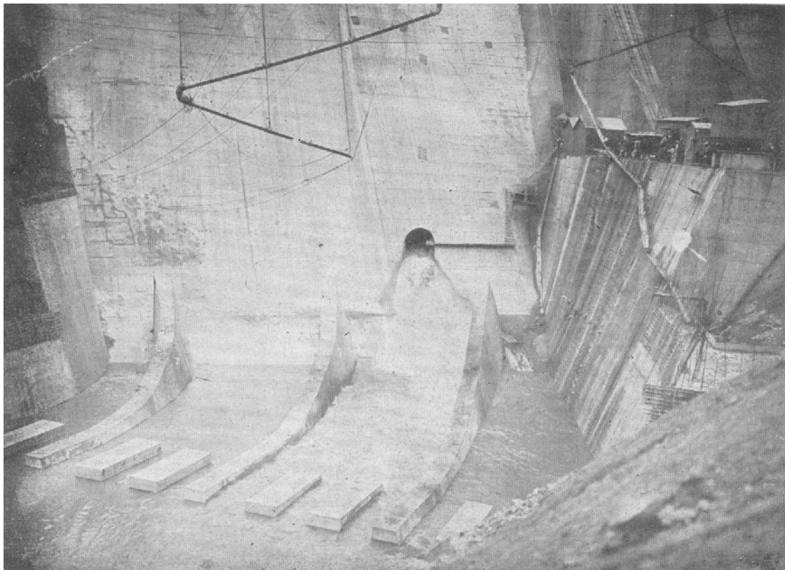
Barrage de l'oued Beth, radier aval en cours d'achèvement (1933)
