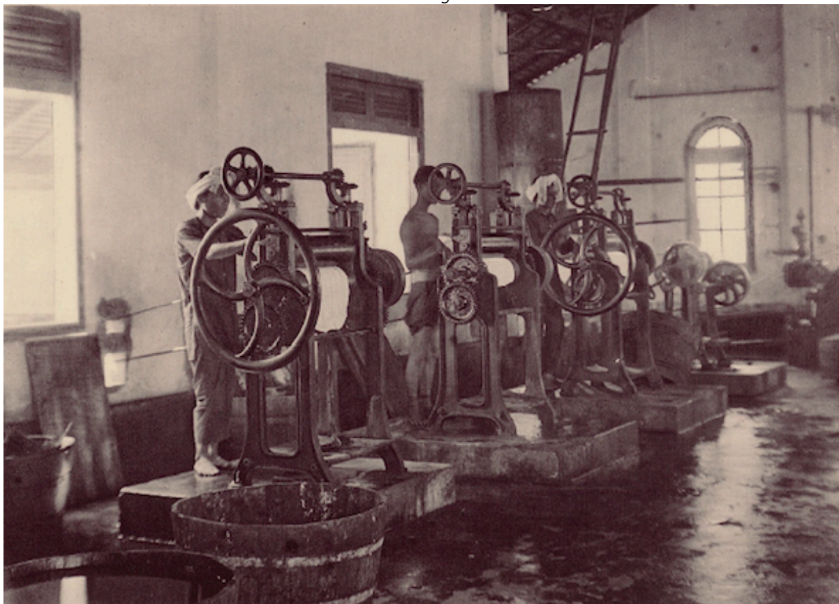
Planche 57. — Préparation des feuilles au laminoir
